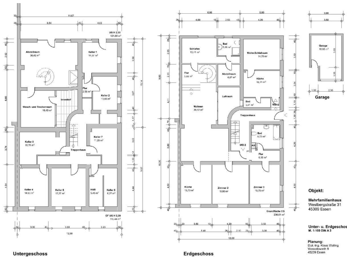
Grundriss Unter- und Erdgeschoss
