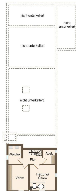
Grundriss KG
