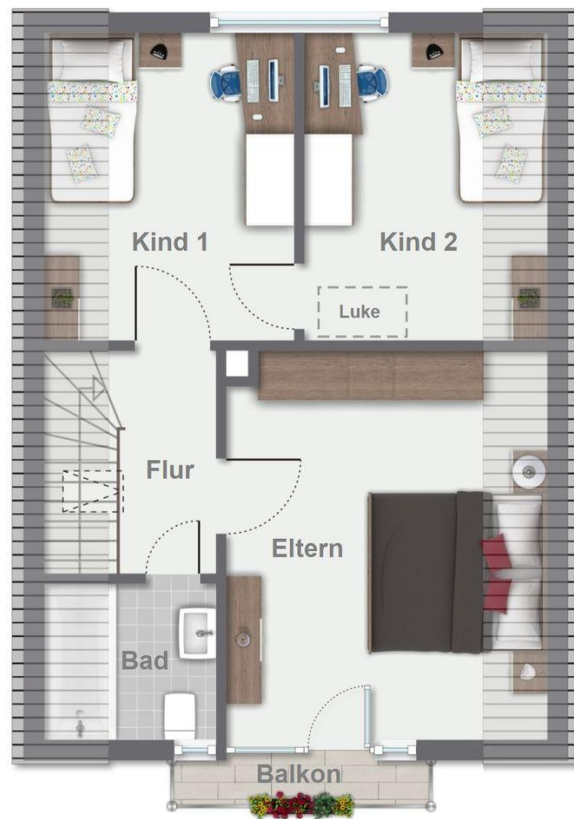
Grundriss Dachgeschoss
