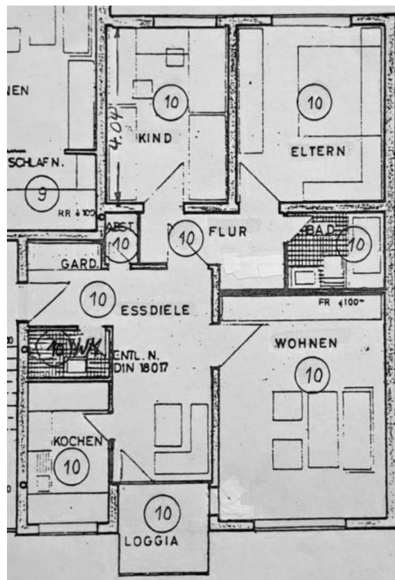
Grundrisskizze
