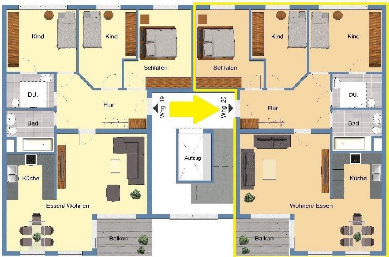
Haus 8 -Grundriss 2. OG
