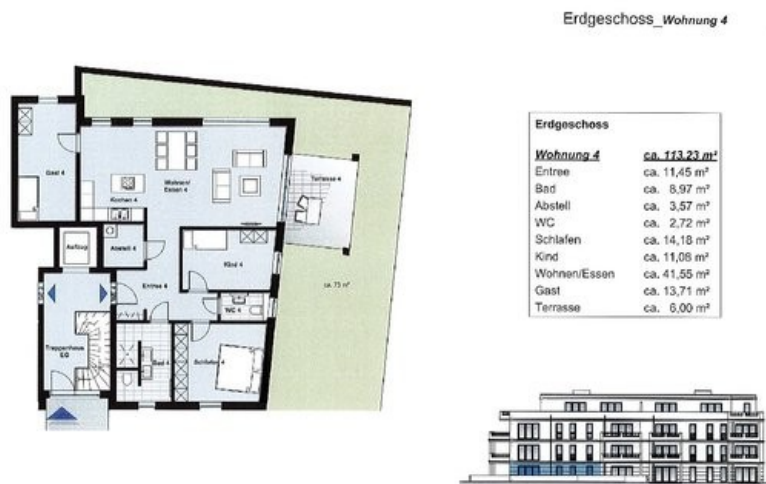
Grundriss
